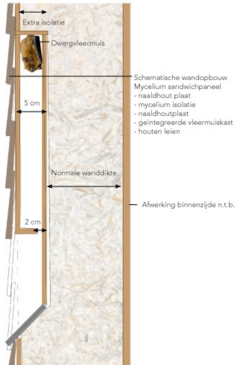
Wandopbouw met vleermuiskast
